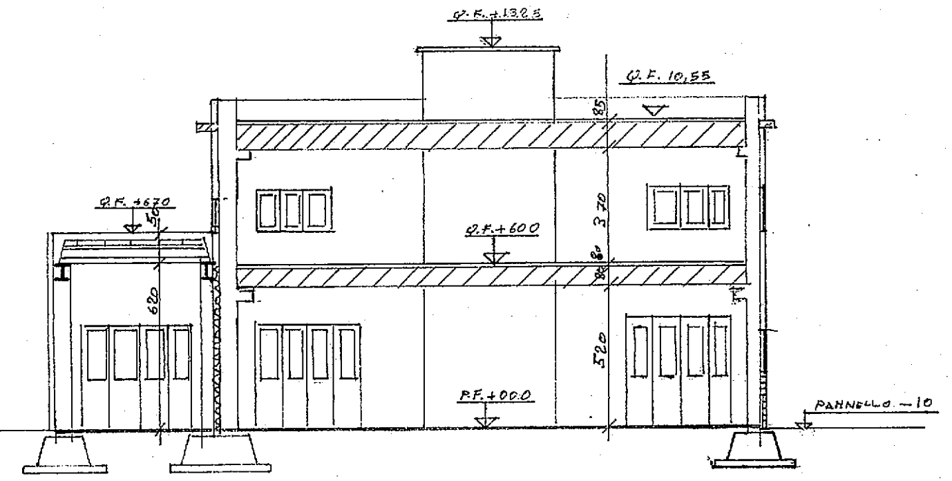
SEZIONE LONGITUDINALE FABB. F-E
