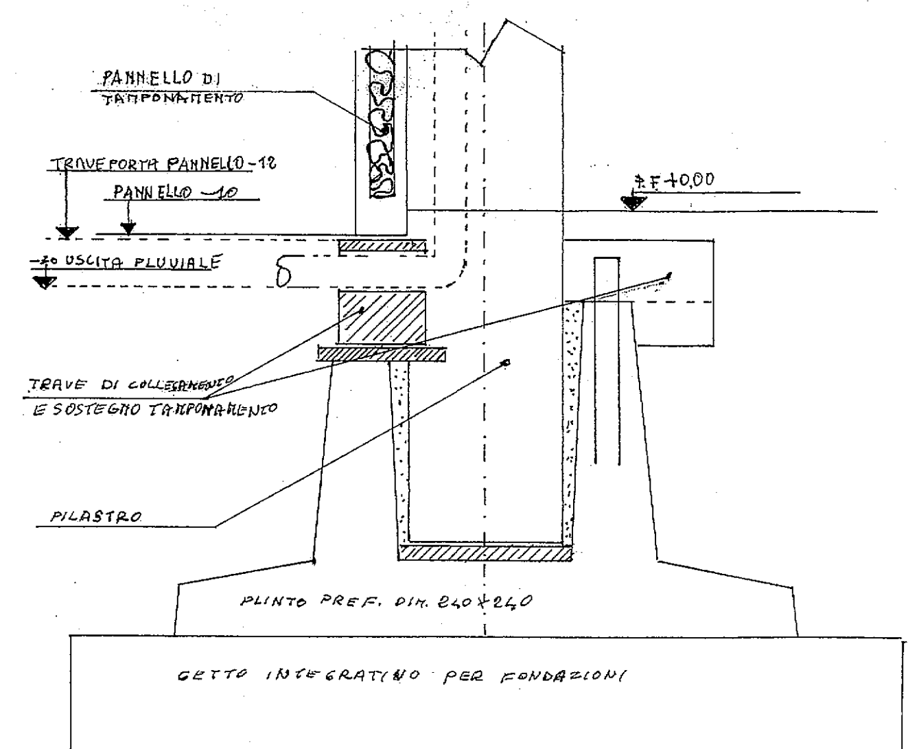
PLINTO DI FONDAZIONE SCALA 1:20
